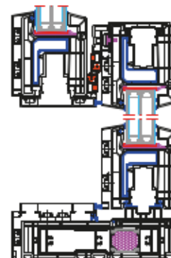
Przekrój poziomy przez skrzydło czynne
