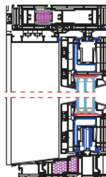
Przekrój pionowy przez skrzydło czynne
