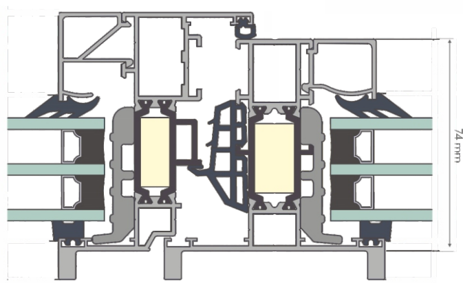
PRZEKRÓJ PRZEZ SŁUPEK TM 74HI INDUSTRIAL
