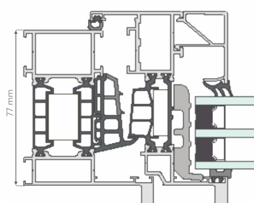
PRZEKRÓJ PRZEZ OKNO TM 77HI INDUSTRIAL
