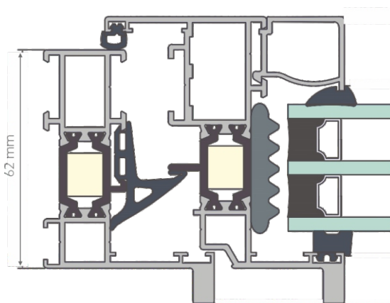
PRZEKRÓJ PRZEZ OKNO TM 62HI INDUSTRIAL
